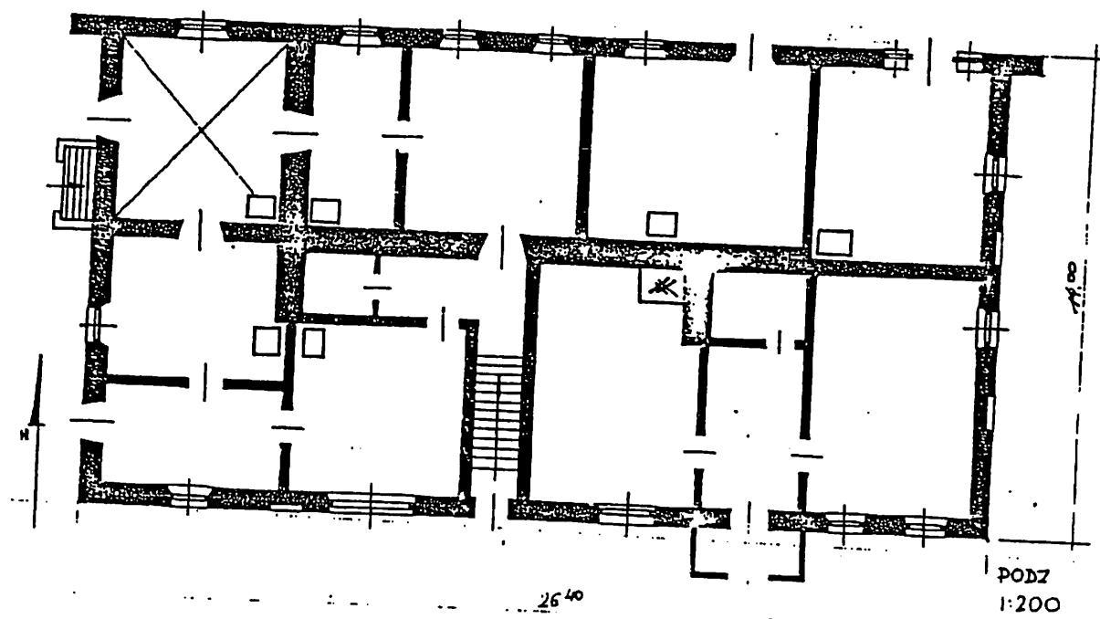
Rzuty budynków przy ul. Warszawskiej nr 1.
